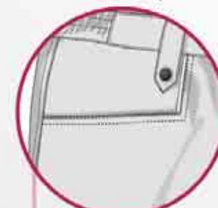
7-BOLSILLO CON VIVO
