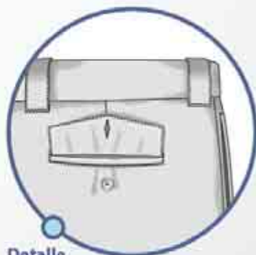
Detalle BOLSILLO TRASERO con vivo, ojal, botón y tapeta en punta
